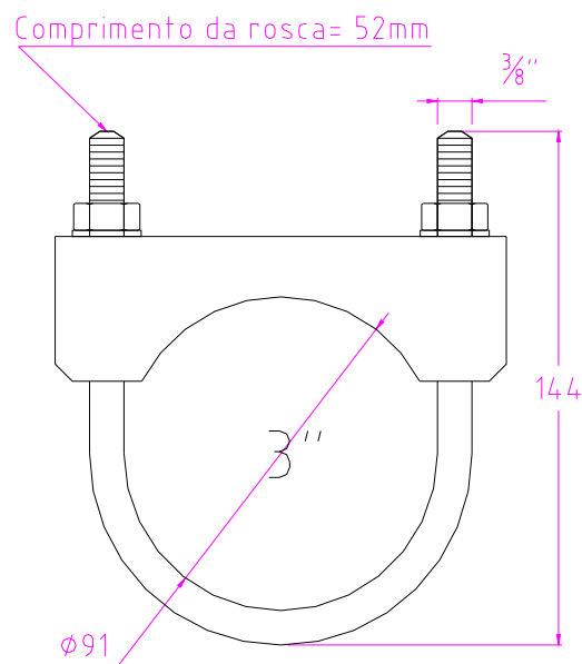
Desenho com medidas (sem escala)
