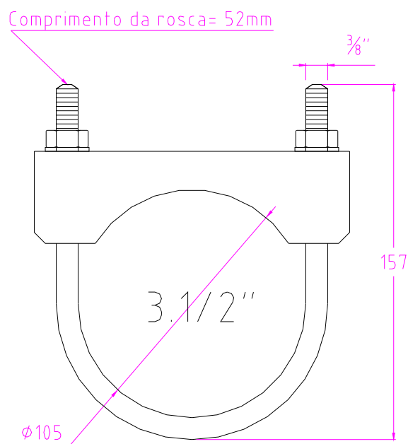
Desenho com medidas (sem escala)
