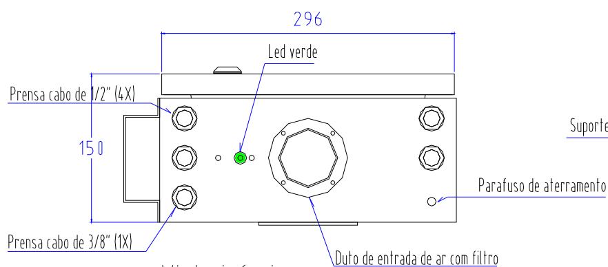
Vista inferior
