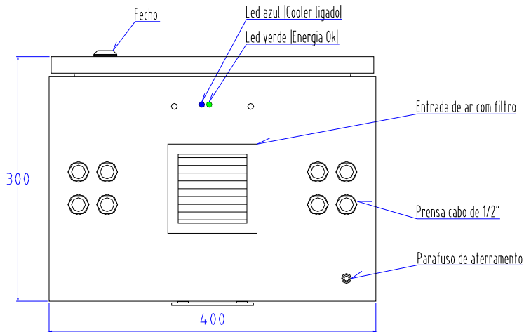
Vista inferior
